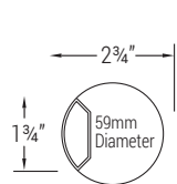
ROUND GROMMET (G1)
